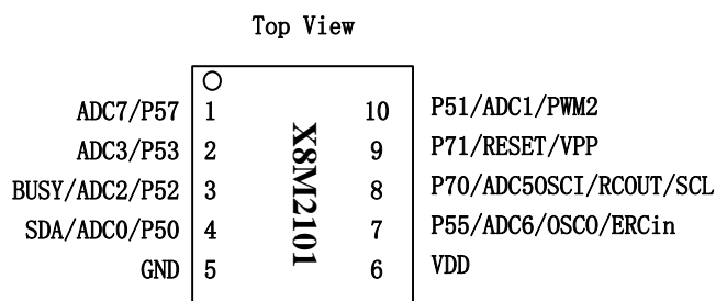
X8M2101-10PIN 脚位图
