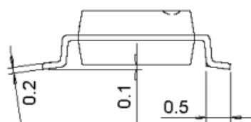
SOP14 封装尺寸
