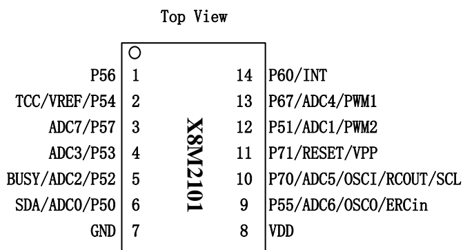
X8M2101-14PIN 脚位图
