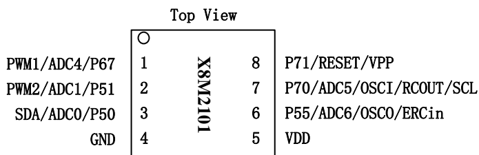
X8M2101-8PIN 脚位图
