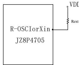
内部电容振荡器模式电路
