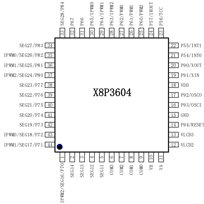
X8P3604-44PIN 脚位图
