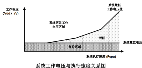
系统工作电压与执行速度关系图
