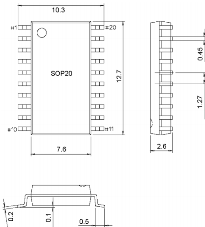
SOP20 封装尺寸
