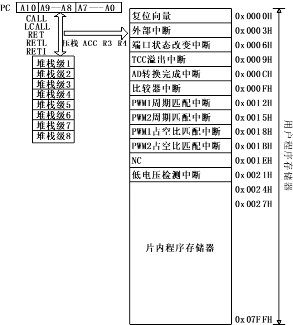
程序存储器区结构图
