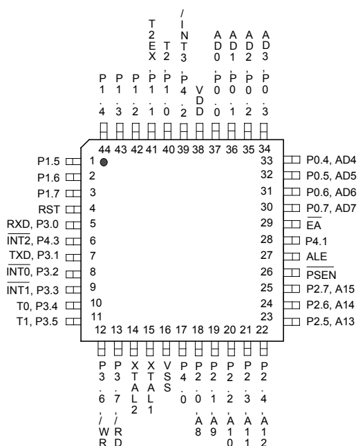
44-Pin QFP (W78E54BF)
