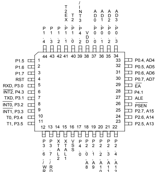
44-Pin QFP (W78E516BF)
