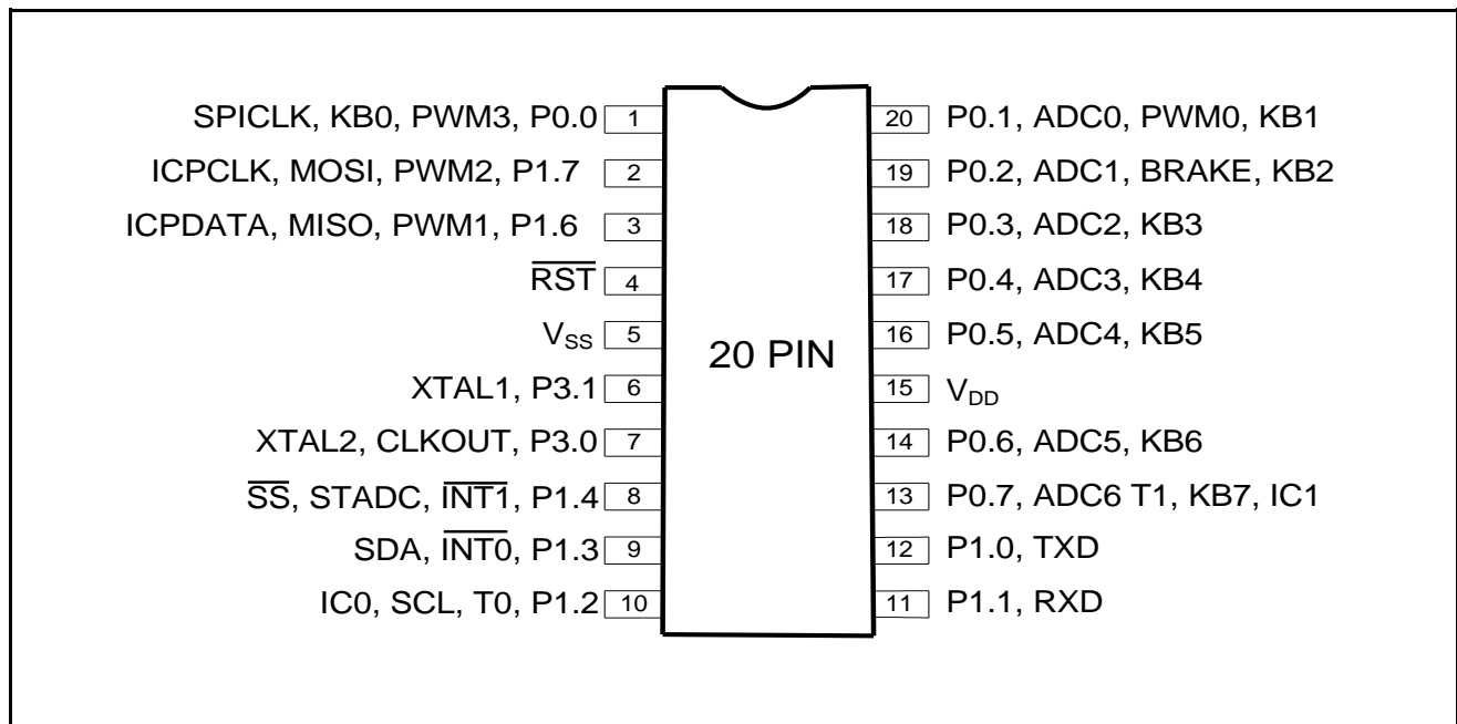
图5-2. TSSOP20 管脚分配
