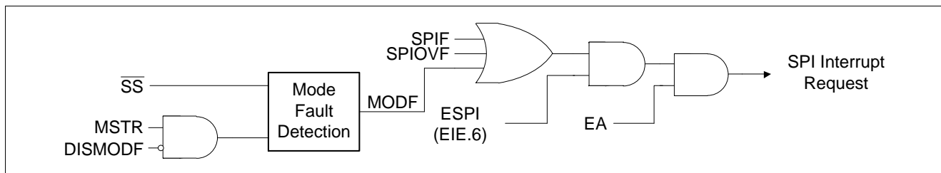
图13-8. SPI 中断请求
