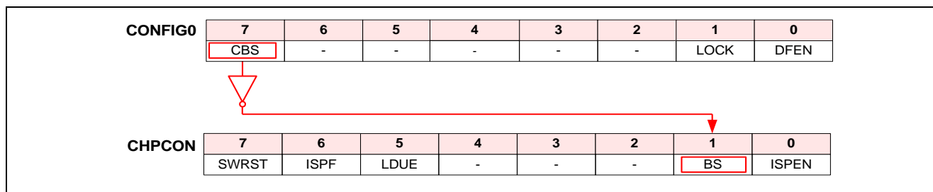
图25-1. 配置位0 复位重载（软件复位除外）
