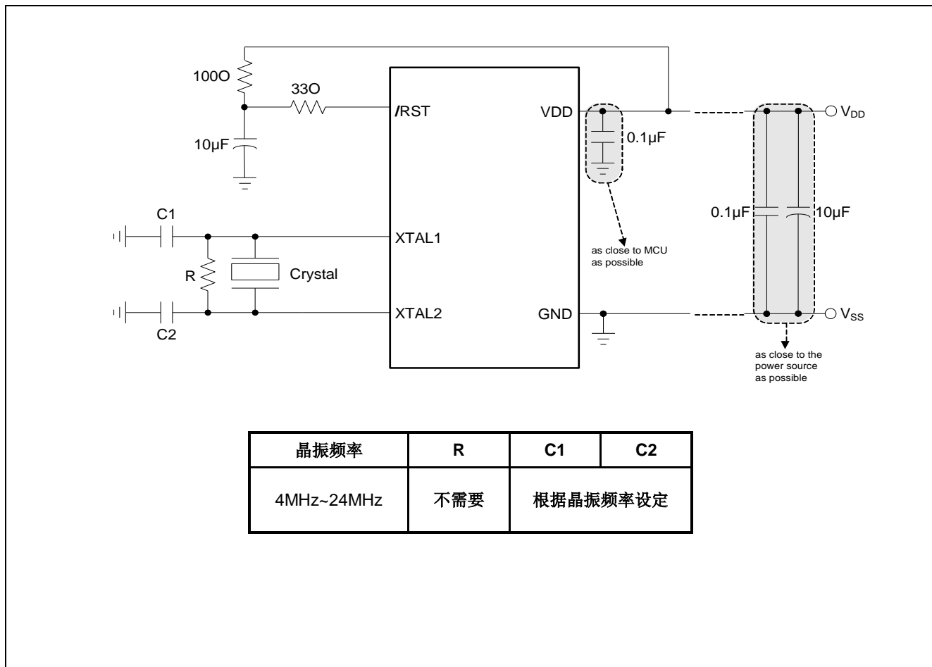
图29-1. 增加抗干扰性能建议电路
