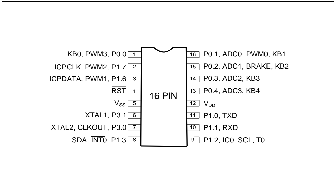
图5 - 3. SOP 16管脚分配
