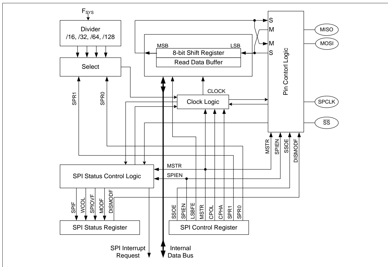
图13-1. SPI 模块结构图
