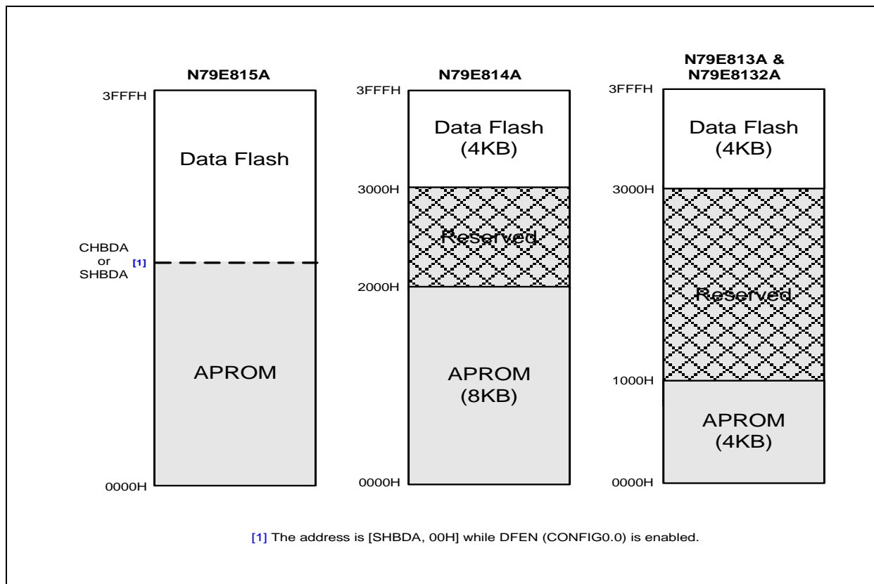
图6-2. N79E815A/814A/8132A 数据存储器
