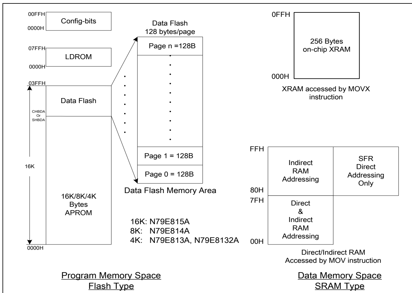
图6-1 N79E815A/814A/8132A 内存结构图
