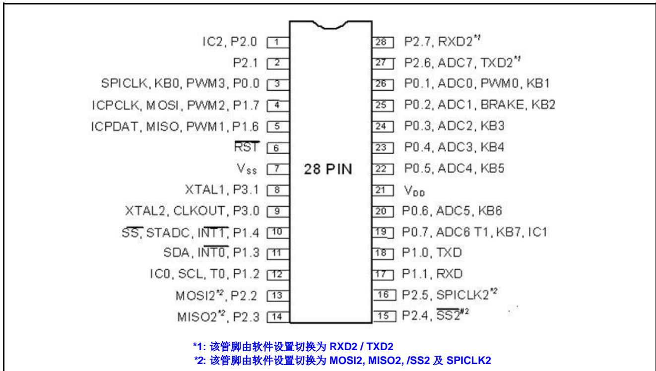
图5-1. TSSOP28 管脚分配图
