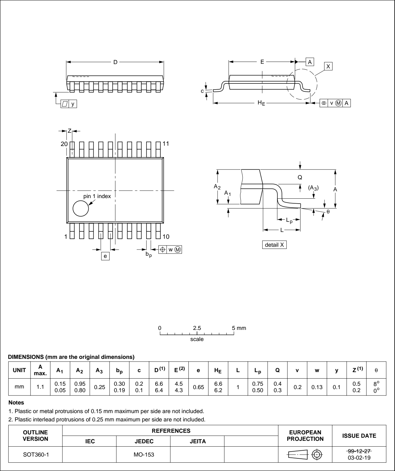
Fig 14. TSSOP20 (SOT360-1).
