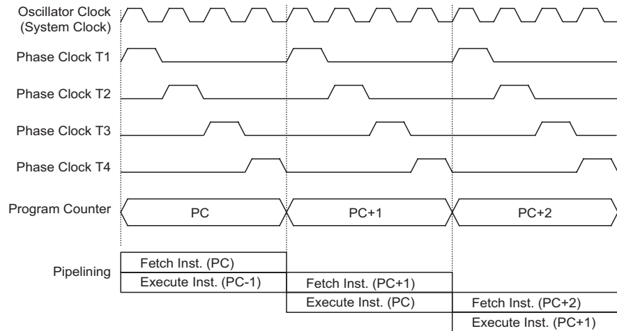
系统时序和流水线
