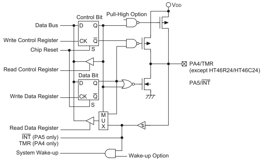
PA4/PA5 输入/输出端口
