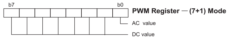
7+1 模式的 PWM 寄存器
