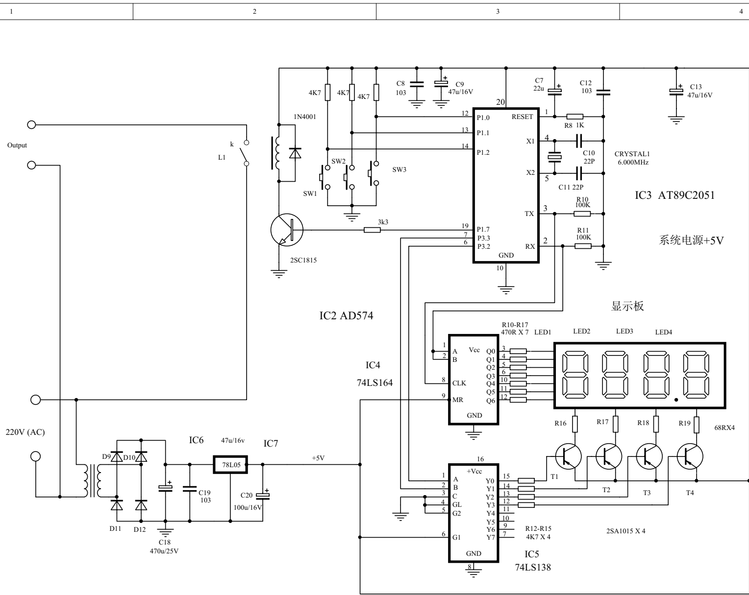
水泵控制器电路图
