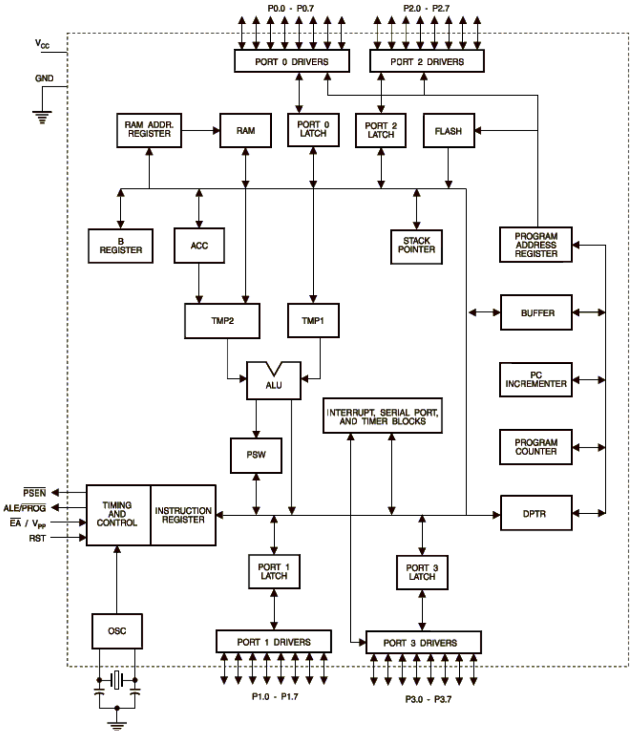
AT89LV51 方框图
